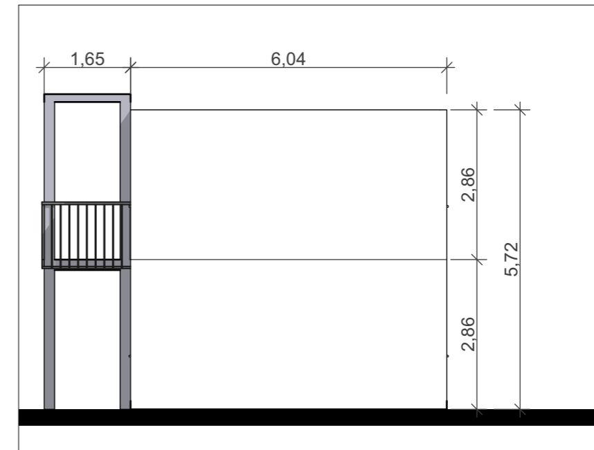
Ansicht West
