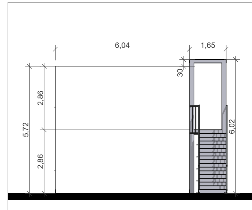
Ansicht Ost
