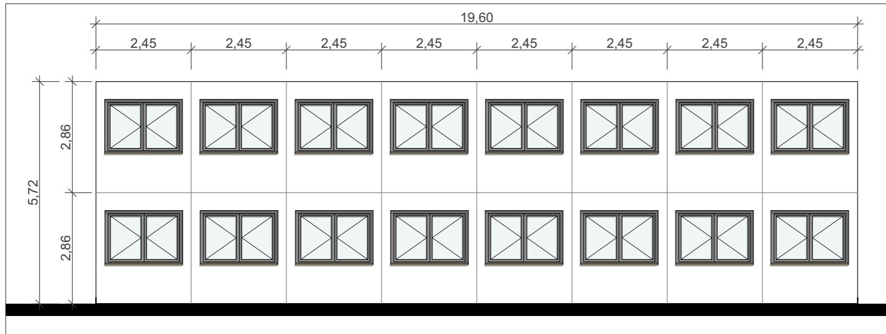
Ansicht Süd
